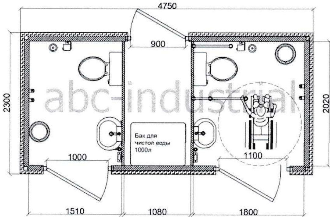
Планировка туалетного модуля "Амстердам" (автономный)
